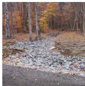
Enrochement - Source : Morin Heights
