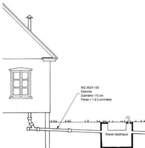
Figure B.5.1 : La conduite d'amenée
