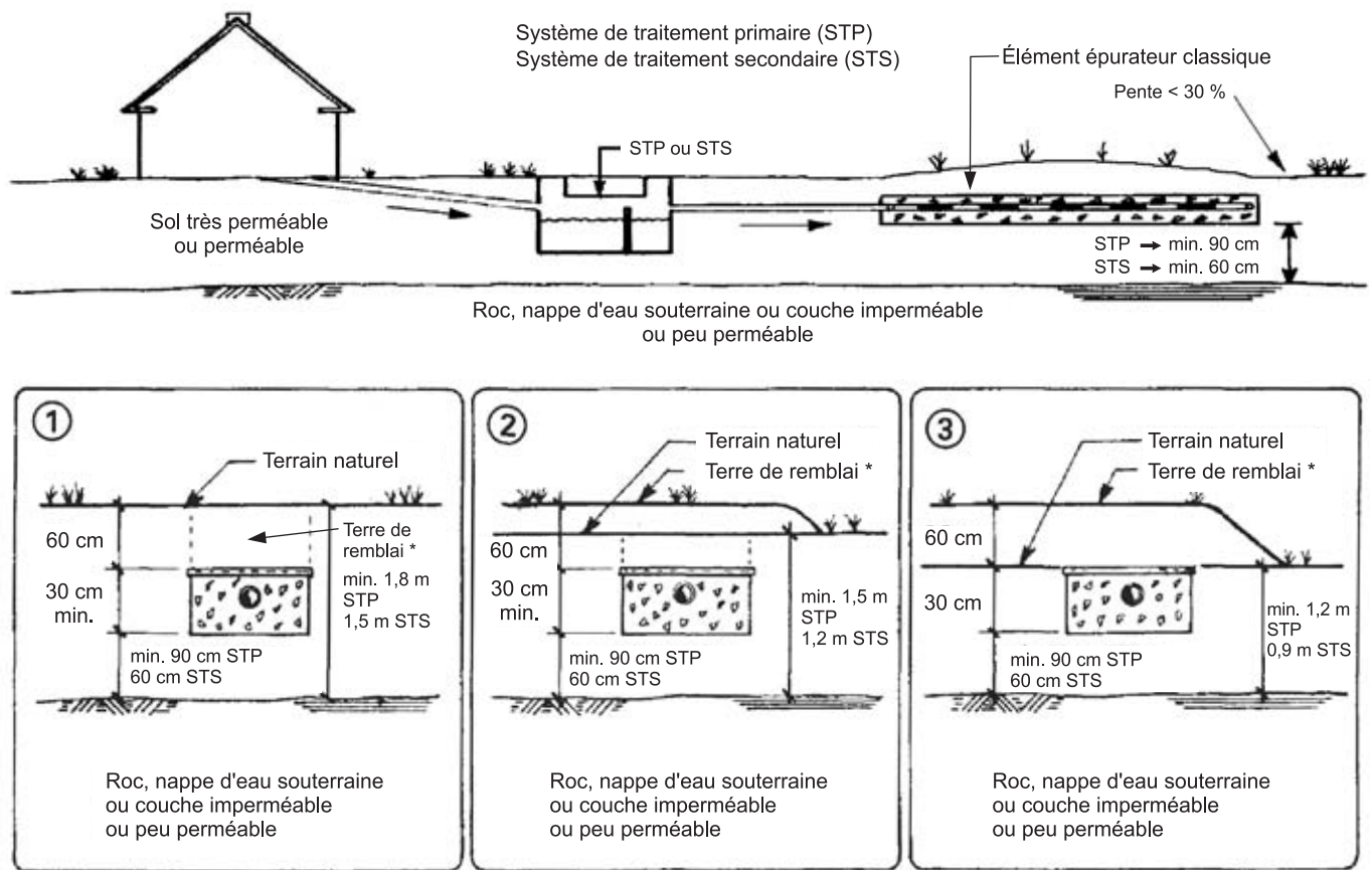
Figure B.9.2 : Le terrain récepteur de l'élément épurateur classique
