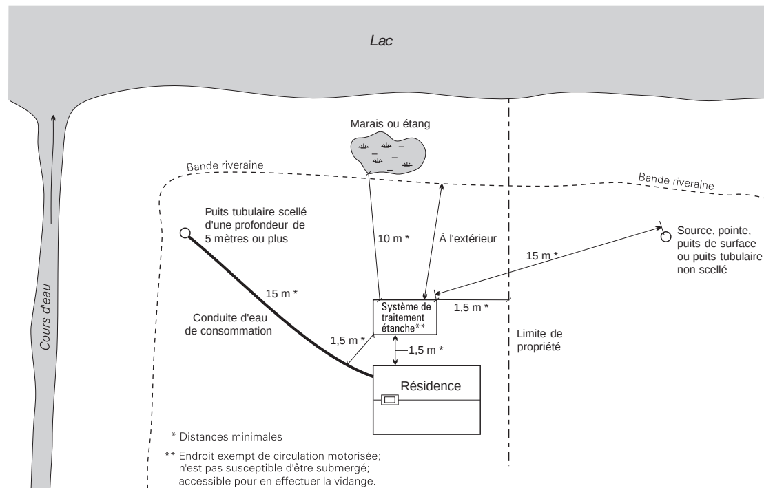
Figure B.4.1 : Localisation d'un système de traitement étanche
