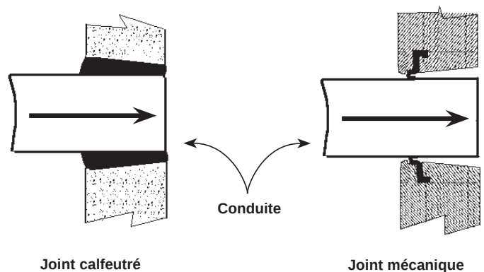
Figure B.5.2 : Détails du raccordement
