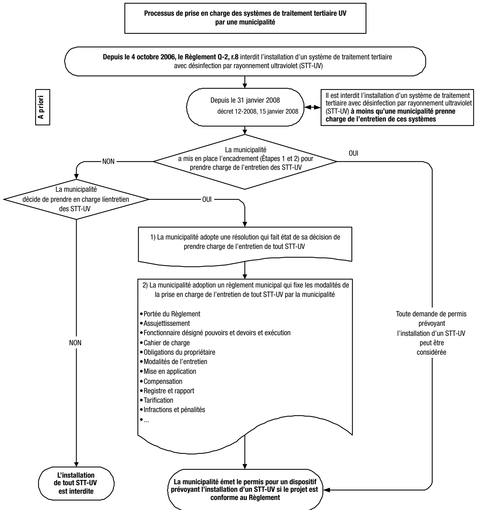
Figure B.19.2 : Processus de prise en charge des systèmes de traitement tertiaire UV par une municipalité
