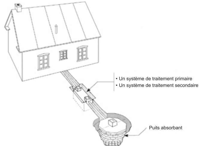
Figure B.11.1 : Le puits absorbant
