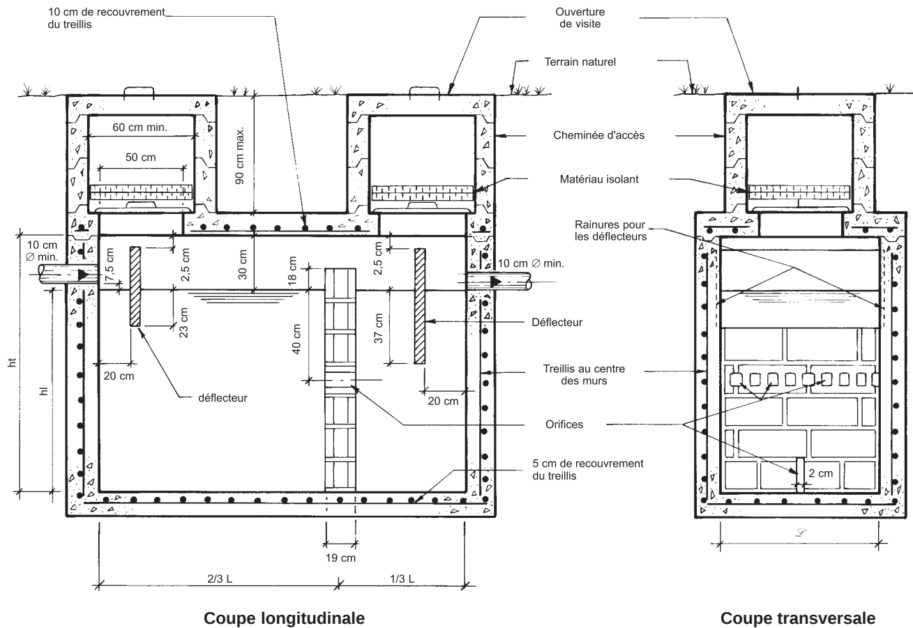
Figure B.6.2 : La fosse septique construite sur place
