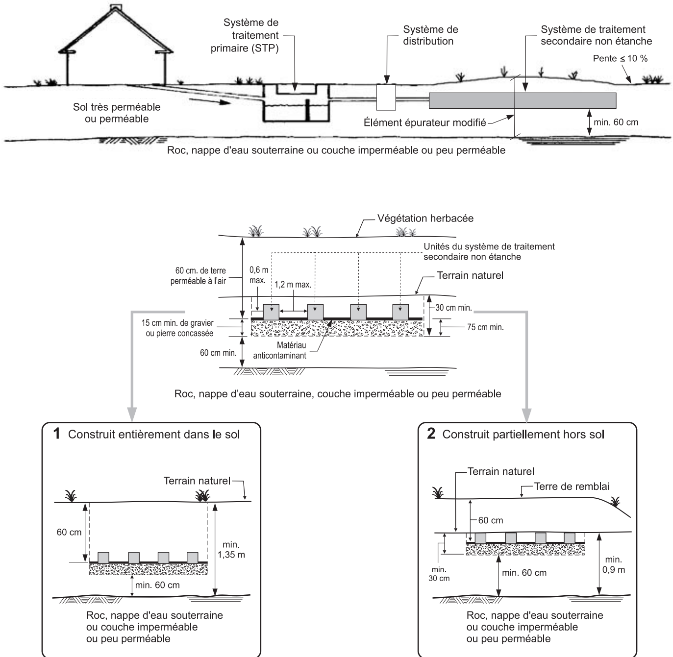
Figure B.10.8 : Détails de construction du lit d'absorption lorsque le système est composé d'unités espacées
