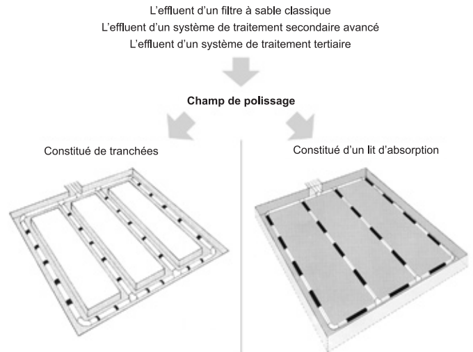
Figure B.20.1 : Le champ de polissage
