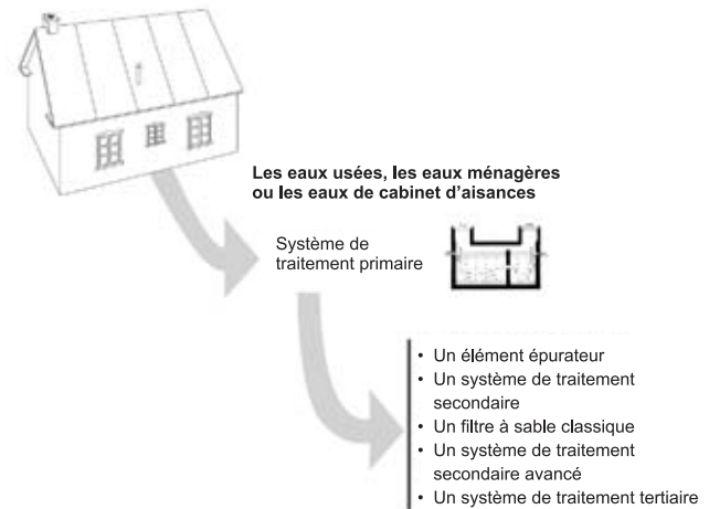
Figure B.6.1 : Cheminement des eaux et de l'effluent d'un système de traitement primaire
